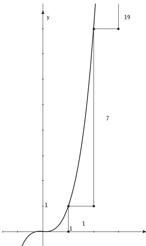
Figura 3 Tratamiento cuantitativo, polinomio y = x^3
