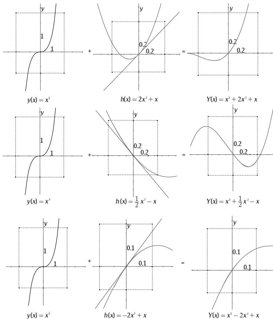
Figura 2 Ejemplos del comportamiento de los términos cuadrático y lineal para el polinomio cúbico ( Y(x)=ax^3 + bx^2 + cx )
