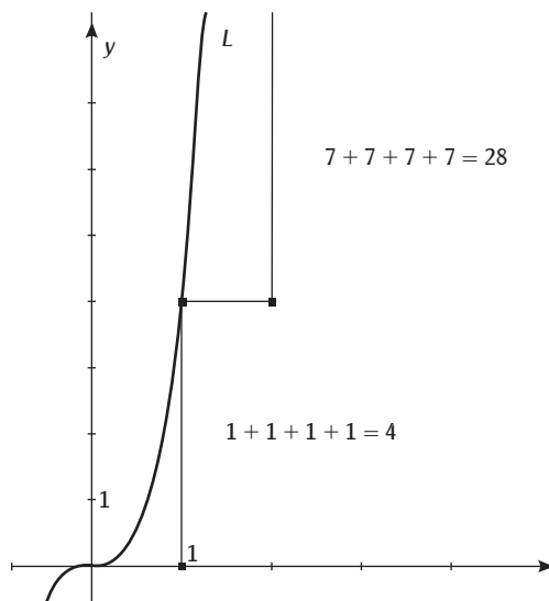
Figura 4 Tratamiento cuantitativo para identificar la secuencia numérica del polinomio cúbico L
