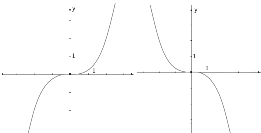
Figura 1 Comportamiento del polinomio cúbico y = ax^3 , ( a > 0 y a < 0 , respectivamente)
