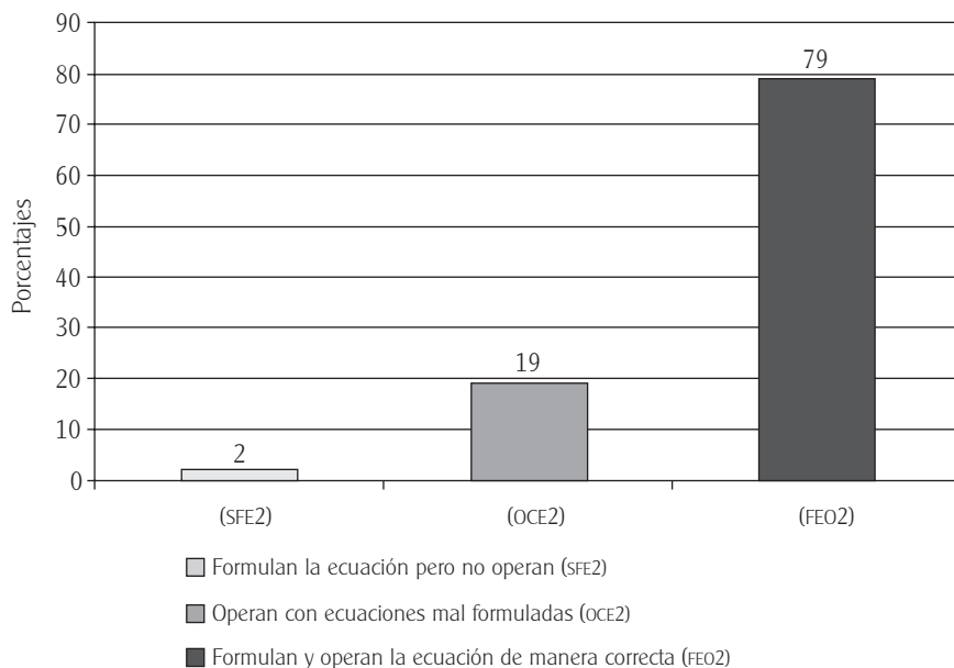
Gráfica 4 Resoluciones algebraicas del problema 2 (N = 52)
