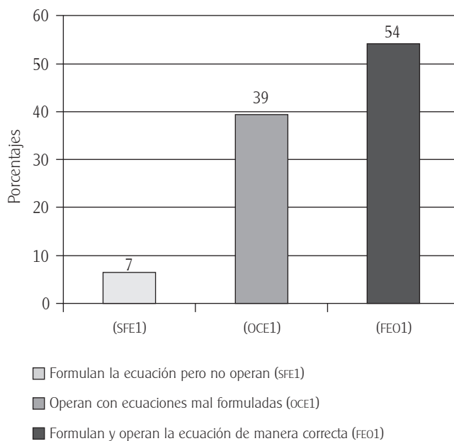
Gráfica 2 Resolución algebraica del problema 1 ( N = 122 )
